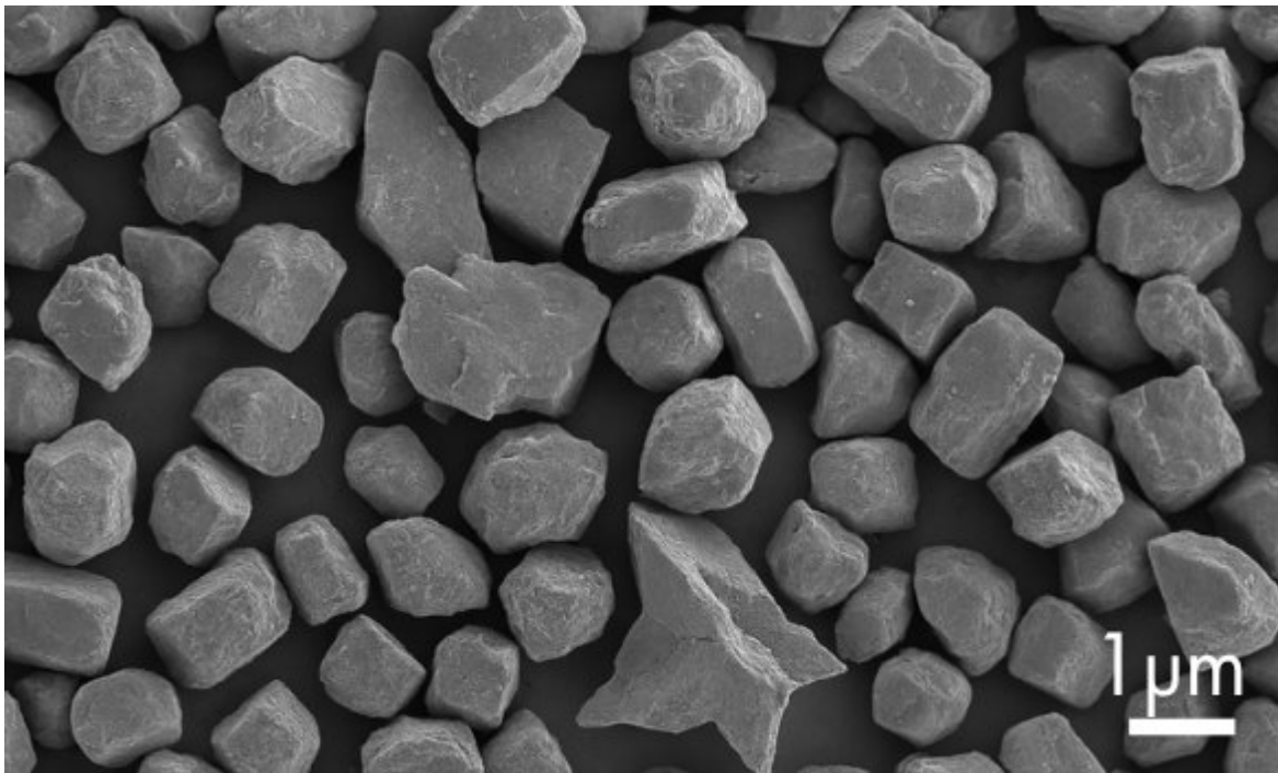
Figuur 1. Microscopisch onderzoek naar bronnen van calciumcarbonaat: (links) gewoon gemalen calciumcarbonaat (Bron: © Sirris), (rechts) circulair calciumcarbonaat uit eierschalen (Bron: © EGGXPRT).
