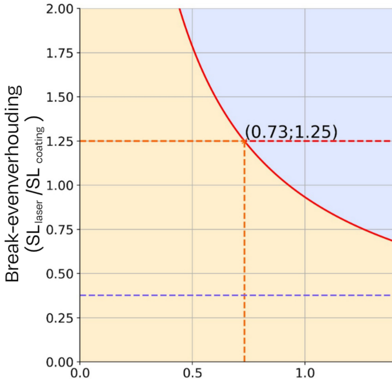
Figuur 2. Break-even van de 'single score' Product Environmental Footprint (PEF), die het effect van de gebruiksduur van beide oppervlaktebehandelingen op de milieu-impact aantoon.
